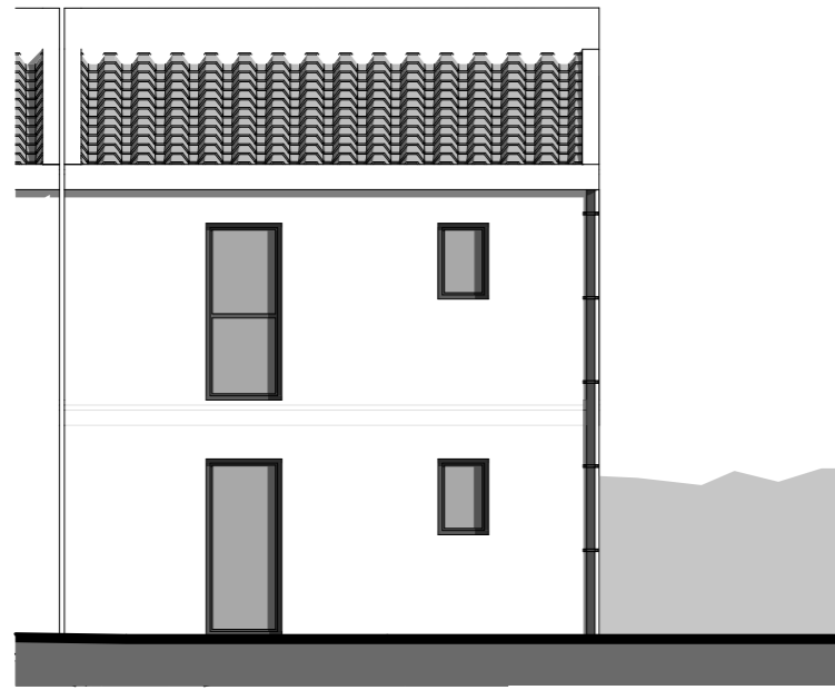
Façade NORD 1 : 100
