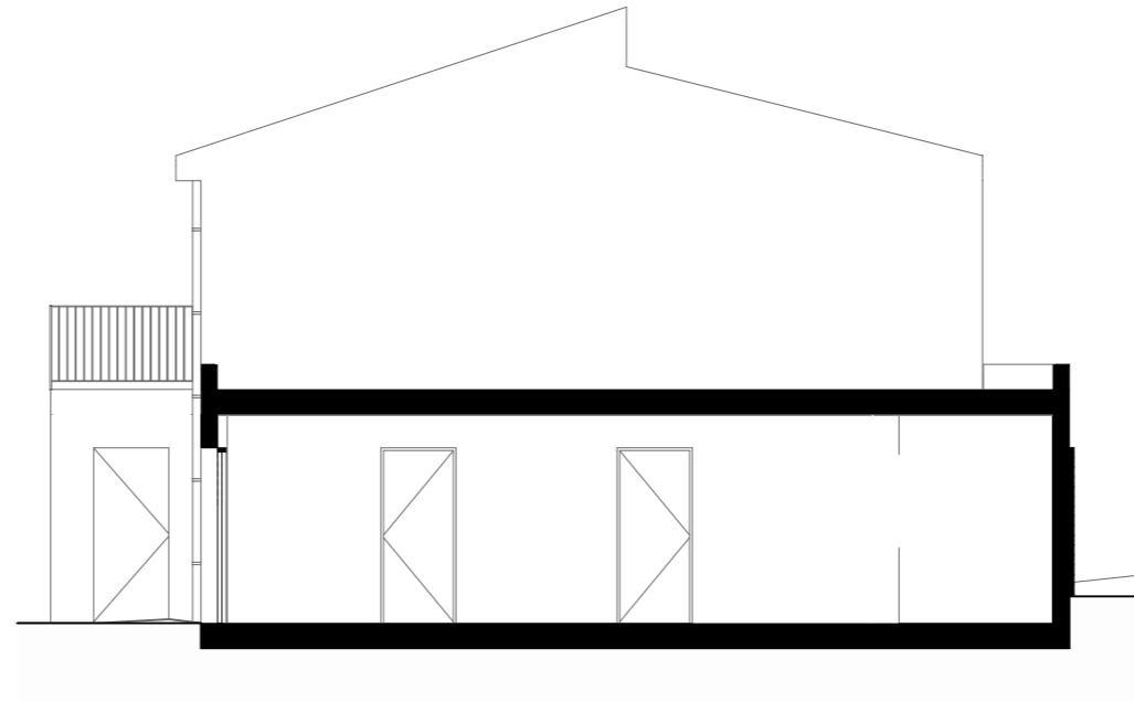
Façade OUEST 1:100
